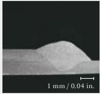
/ Dip-transfer arc I: 185 A, U: 17.6 V
